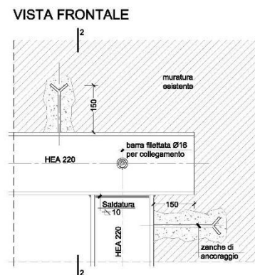
PARTICOLARE "B" 1:10
